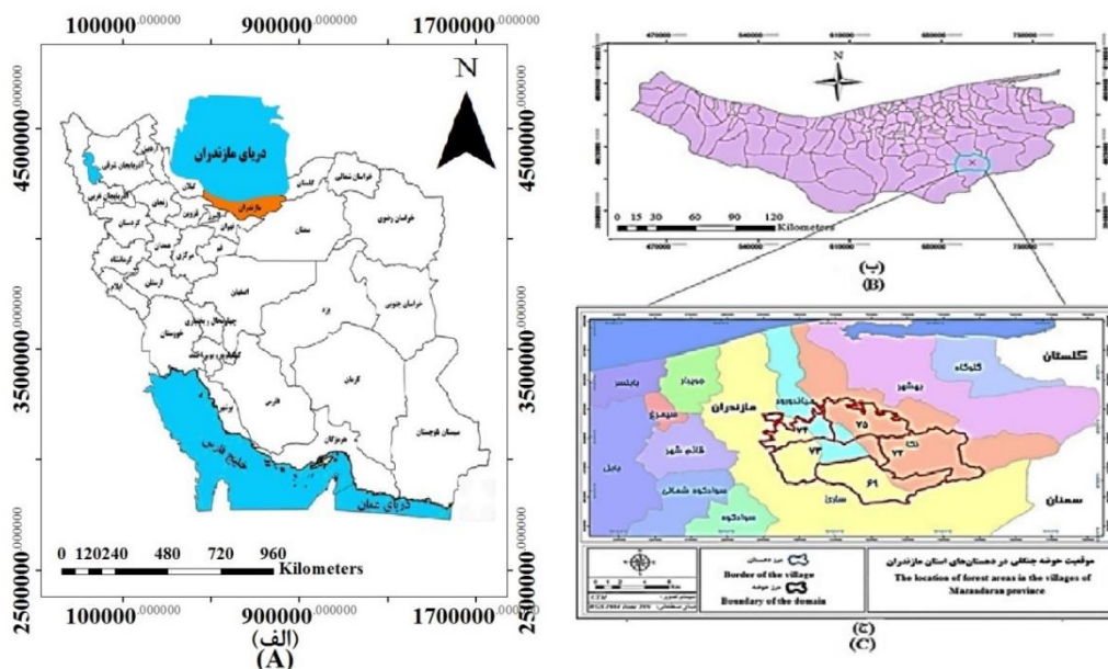
شکل ۱- موقعیت منطقه مورد مطالعه به‌ترتیب در: (الف) کشور ایران، (ب) استان مازندران و (ج) حوزه‌های آبخیز رودخانه تجن مورد مطالعه Figure 1. The location of the studied area in: A) Iran, B) Mazandaran province and C) Studied Tajan river watersheds.
