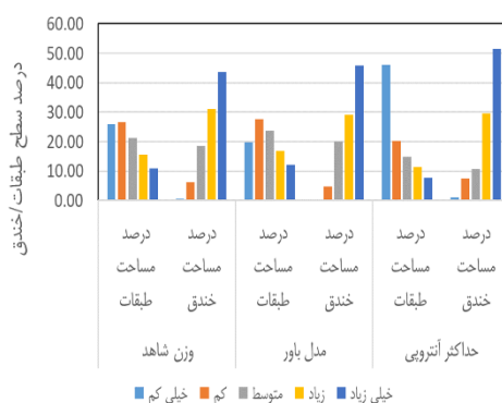
شکل ۶- سطح سلول هسته در طبقات حساسیت به فرسایش آب‌کندی در حوزه آبخیز سد مارون Figure 6. The seed core area indexes in gully erosion susceptibility classes in the Maroon Dam watershed
