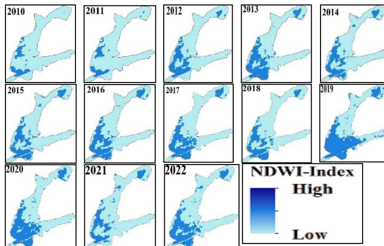
شکل ۴- تصاویر ماهواره‌ای مودیس شاخص NDWI تالاب شادگان در دوره ۱۳ ساله Figure 4. MODIS Satellite Images of the NDWI Index for the Shadegan Wetland over a 13-Year Period
