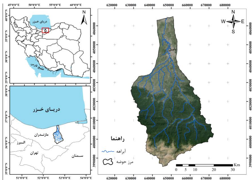
شکل ۱- موقعیت جغرافیایی حوضه آبخیز بابلرود در ایران و استان مازندران Figure 1. Geographic Location of Babilrood watershed in Iran and Mazandaran Province
