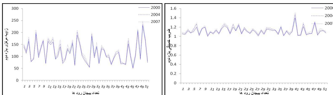
شکل ۱۰- مقایسه ضریب خمیدگی پیچان های بازه دوم.
