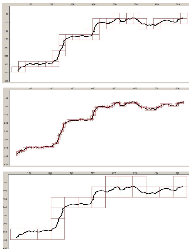
شکل ۶- نحوه محاسبه بعد رودخانه به روش بعد شمارش خانه با تغییر مقیاس (بازه اول محدوده مورد مطالعه از تصویر لندست ۲۰۰۴).
