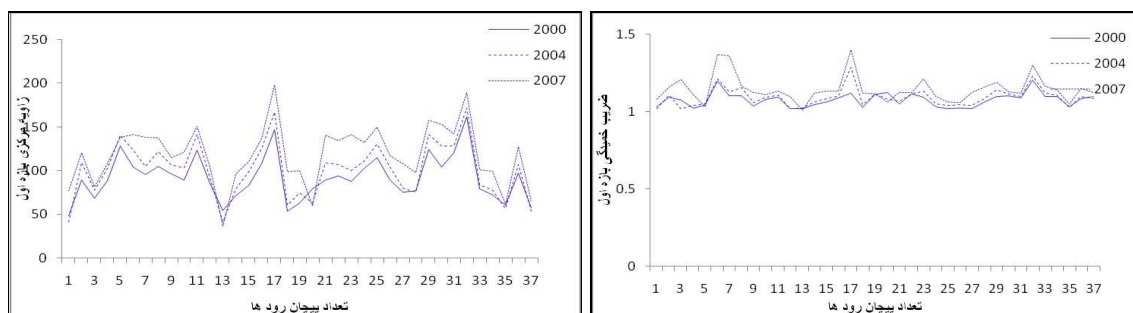
شکل ۸- مقایسه ضریب خمیدگی پیچان های بازه اول.
