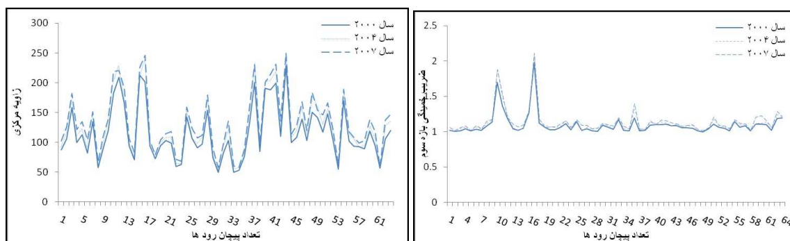
شکل ۱۲- مقایسه ضریب خمیدگی پیچان های بازه سوم.
