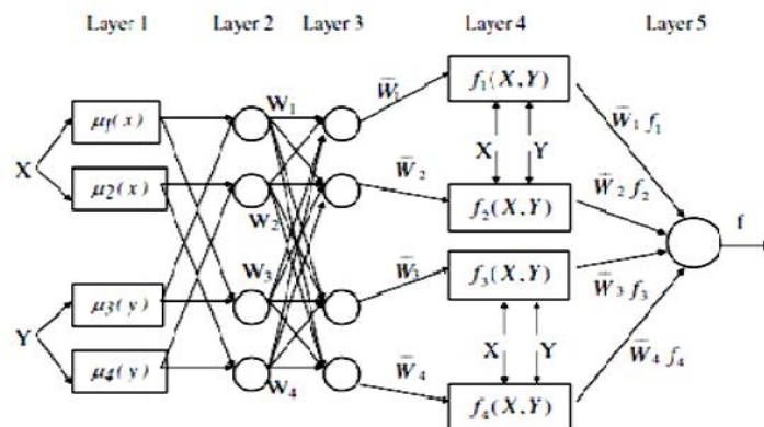
شکل ۲- شمای ساده‌ای از مدل ANFIS
