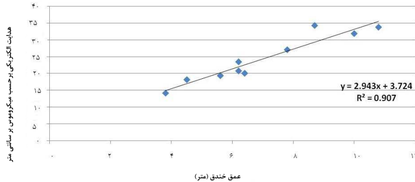
شکل ۴- رابطه بین عمق خندق با مقدار هدایت الکتریکی خاک.
