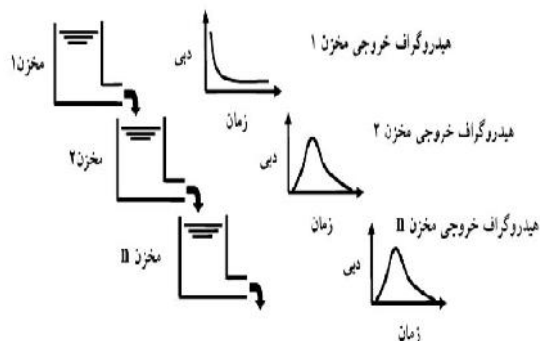
شکل ۲- رفتار آبخیز به عنوان آبشاری از مخزن خطی متوالی (۱۳)
