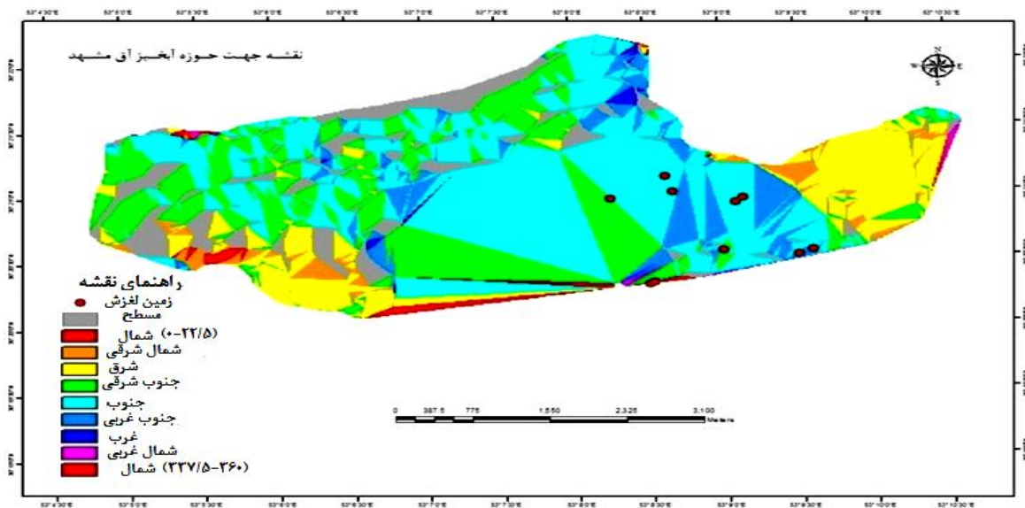
شکل ۲- نقشه جهت حوزه آق مشهد
