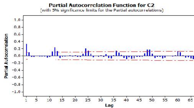
شکل ۳- نمودار مربوط به خودهمبستگی جزئی داده‌های رسوب تبدیل شده
