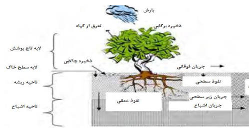
شکل ۶- اجزای سیستم هیدرولوژیک حوزه در مدل WetSpa Figure 6. The components of the hydrological system in the WetSpa model
