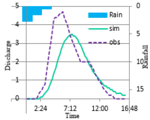
شکل ۱۱- دبی مشاهده‌ای و شبیه‌سازی شده در رویداد ۹۱/۱۰/۰۵ در حوزه یکپارچه کوه‌سوخته Fig. 11. Observational and simulated discharge in the event of 2012/12/25 in the Lumped Kohsukhteh watershed .
