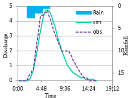
شکل ۱۰- دبی مشاهده‌ای و شبیه‌سازی شده در رویداد ۹۱/۱۰/۰۵ در حوزه نیمه‌توزیعی کوه‌سوخته-زیر حوزه ۳ Fig. 10. Observational and simulated discharge in the event of 2012/12/25 in the semi-distributive Kohsukhteh watershed-sub-catchment 3
