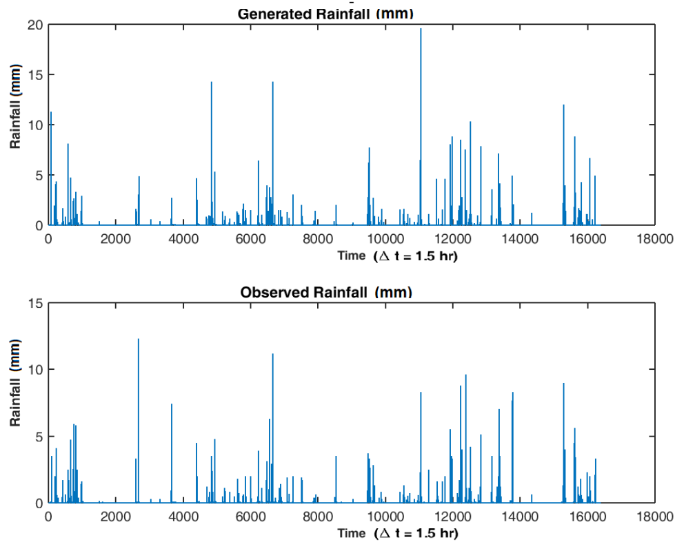
شکل ۷- نمودار سری زمانی بارش‌های مشاهده‌ای (پایین) و محاسباتی (بالا) ایستگاه خودکار دندی در مقیاس ۱/۵ ساعته Figure 7. Graph of both the observed (lower) and the generated (upper) time series of rainfalls of Dandi automatic station in 1.5-hour scale
