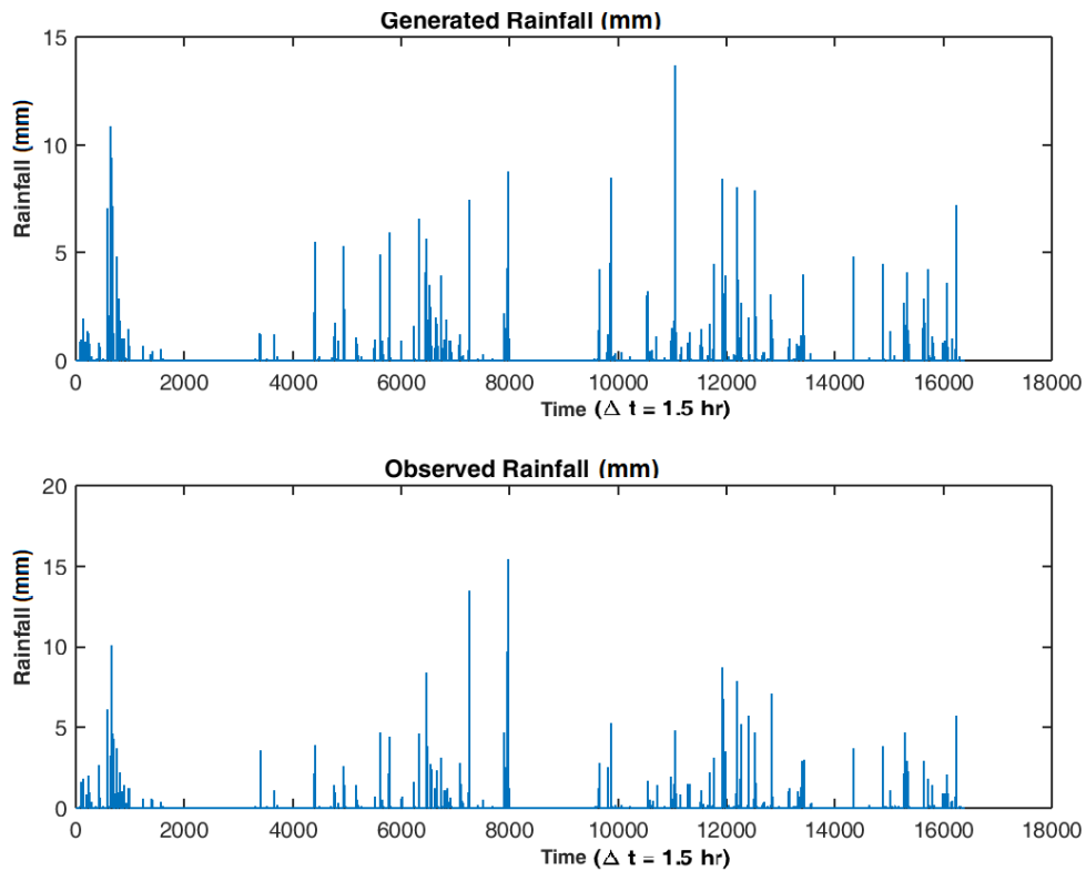
شکل ۶- نمودار سری زمانی بارش‌های مشاهده‌ای (پایین) و محاسباتی (بالا) ایستگاه سینوپتیک زنجان در مقیاس ۱/۵ ساعته Figure 6. Graph of both the observed (lower) and the generated (upper) time series of rainfalls of Zanjn synoptic station in 1.5 hour scale
