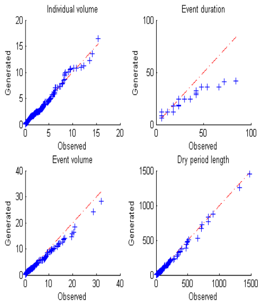
شکل ۹- نمودار چندکی مقادیر بارش منفرد (Individual)، طول دوره‌های تر (Event duration)، مقادیر بارش دوره‌های تر (Event volume) و طول دوره‌های خشک (Dry period duration) در مقیاس‌های مختلف ایستگاه خودکار دندی Figure 9. The quantile-quantile plots for individual values, wet events durations, wet events volumes, and dry period durations in different time scales for Dandi automatic station
