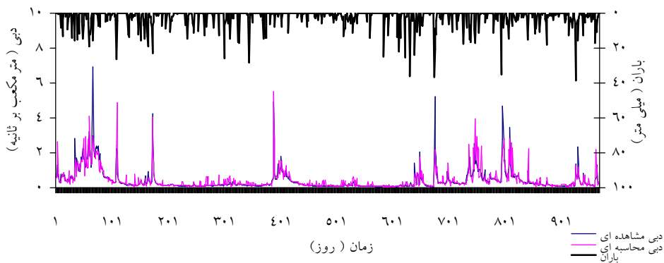
شکل ۴- دبی روزانه مشاهده‌ای و شبیه‌سازی شده شبکه عصبی مصنوعی برای دوره آزمون.
