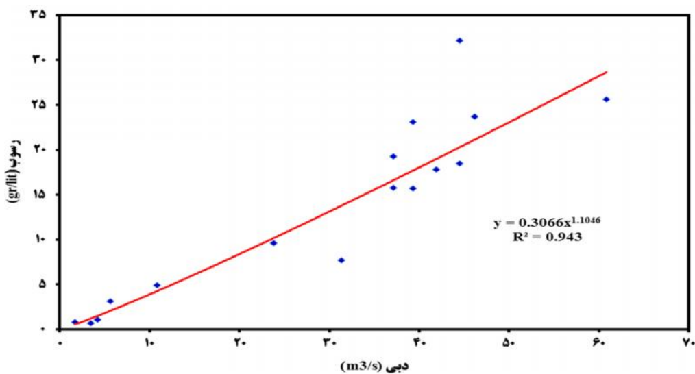
شکل ۱۴- منحنی سنجه رسوب زیرحوزه ۲.
