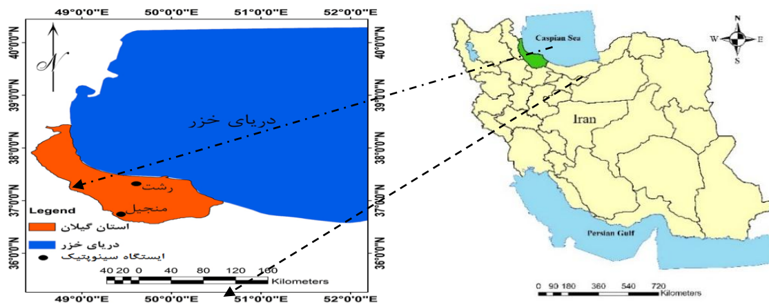
شکل ۱- موقعیت ایستگاه‌های سینوپتیک مورد مطالعه Figure 1. The study area Location
