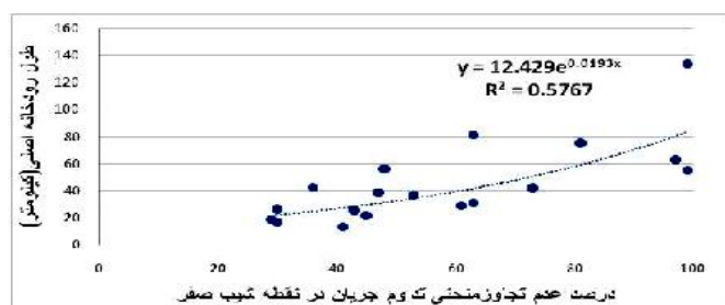
شکل ۴-۲- رابطه درصد عدم تجاوز در نقطه شیب صفر منحنی با طول رودخانه اصلی Figure 4-2. Relationship between exceedance value at the point of zero slope with the main river length
