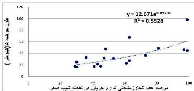
شکل ۴-۴- رابطه درصد عدم تجاوز در نقطه شیب صفر منحنی با طول حوزهها Figure 4-4. Relationship between exceedance value at the point of zero slope with the Catchment length
