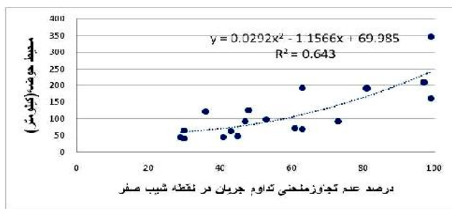
شکل ۴-۱- رابطه درصد عدم تجاوز در نقطه شیب صفر منحنی با محیط حوزهها Figure 4-1. Relationship between exceedance value at the point of zero slope with catchment perimeter
