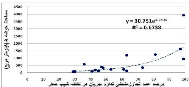
شکل ۴-۳- رابطه درصد عدم تجاوز در نقطه شیب صفر منحنی با مساحت حوزهها Figure 4-3. Relationship between exceedance value at the point of zero slope with the Catchment area
