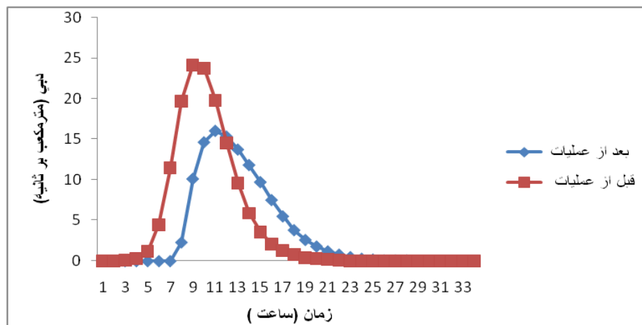
شکل ۷- هیدروگراف خروجی حوزه با دوره بازگشت ۵۰ سال در قبل و بعد از عملیات آبخیزداری Figure 7. Hydrograph of outlet watershed with return periods 50 year in outlet watershed before and after watershed management operations
