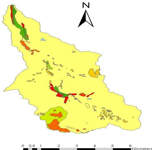
شکل ۲- نقشه CN حوزه هفتان بعد از عملیات آبخیزداری Figure 2. CN map of the Haftan catchment after watershed management operation
