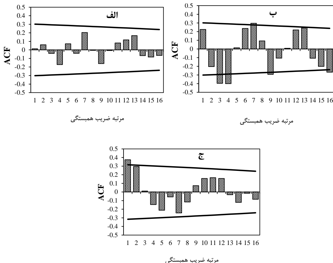
شکل ۵- نمودار تابع خود همبستگی سری‌های زمانی الف (دبی)، ب (بارندگی) و ج (دما) ایستگاه آرازکوسه Figure 5. A time series graph autocorrelation function, A (discharge), B (rainfall) and C (temperature) Arazkoseh station
