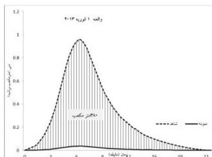
شکل ۲- هیدروگراف سیلاب مشاهداتی حوزه شاهد و نمونه (اول فوریه ۲۰۱۳)
