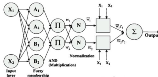
شکل ۲- شبکه CANFIS (۵)
