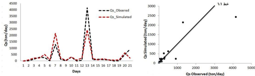
شکل ۵- بار رسوب مشاهده‌ای در مقابل رسوب برآورد شده توسط S3_CANFIS در طول فرآیند آزمون شبکه Figure 5. Observed sediment load versus simulated sediment load by the S3-CANFIS during testing process
