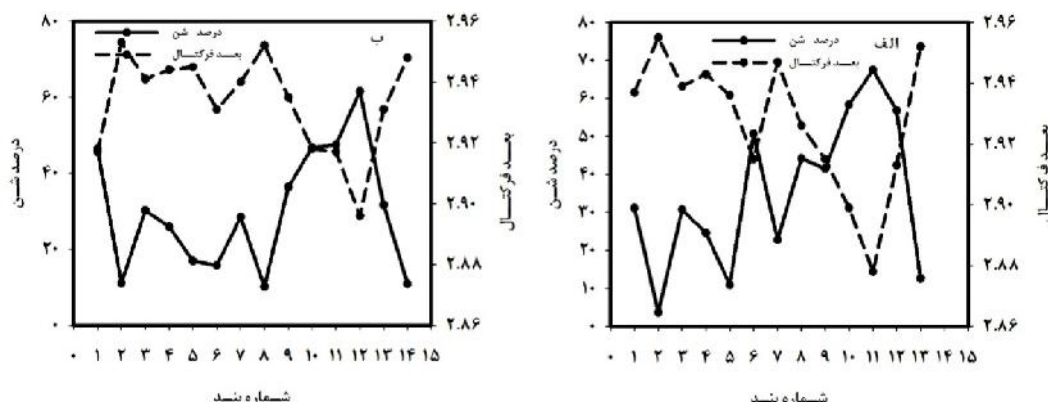
شکل ۳- ارتباط بعد فرکتال (D) با درصد شن در برندهای متوالی در دو عمق ۰-۱۵ (الف) و ۱۵-۳۰ (ب) سانتی متری Figure 3. The relationship between fractal dimension (D) and sand content in successive check dams in depths of 0-15 and 15-30 cm
