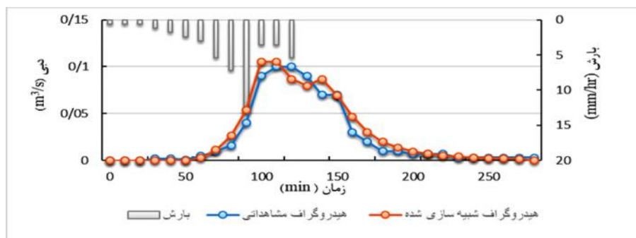
شکل ۷- نتایج واسنجی: هیدروگراف شبیه سازی شده و مشاهداتی برای رگبار مورخ ۱۳۸۹/۱۰/۲۹
