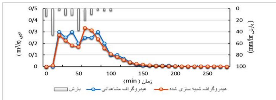
شکل ۶- نتایج واسنجی: هیدروگراف شبیه سازی شده و مشاهداتی برای رگبار مورخ ۱۳۸۹/۱۰/۴
