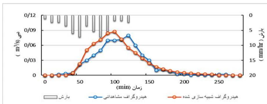
شکل ۸- نتایج واسنجی: هیدروگراف شبیه سازی شده و مشاهداتی برای رگبار مورخ ۱۳۸۹/۱۲/۱۲
