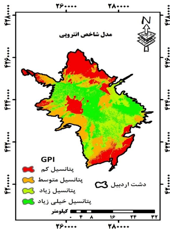
شکل ۵- نقشه پتانسیل منابع آب زیرزمینی دشت اردبیل براساس مدل شاخص آنترופی Figure 5. Groundwater potential map based on Index of Entropy model
