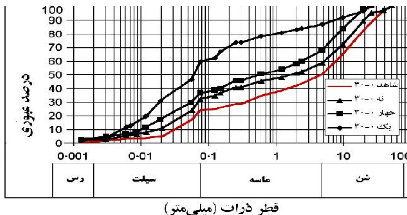
شکل ۹- دانه‌بندی ذرات در عمق ۳۰-۰ سانتی‌متری
