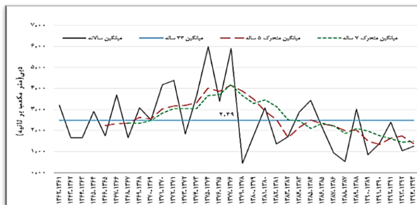
شکل ۴- تغییرات متوسط دبی سالانه ایستگاه کوپال نمره ۳ و میانگین متحرک ۷ و ۱۵ سال‌های طی سال‌های ۱۳۶۱ تا ۱۳۹۴ Figure 4. Yearly variation of water flow rate average and its 7 & 15 years moving averages in Koopal No3 hydrometric station between the years of 1982-2014
