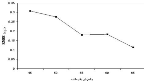
شکل ۳- نمایش تغییرات مقدار متوسط RMSE در مقابل تعداد چاه‌های باقیمانده در شبکه پایش Figure 3. Variation of Mean RMSE vs Number of Remained Wells in monitoring Network
