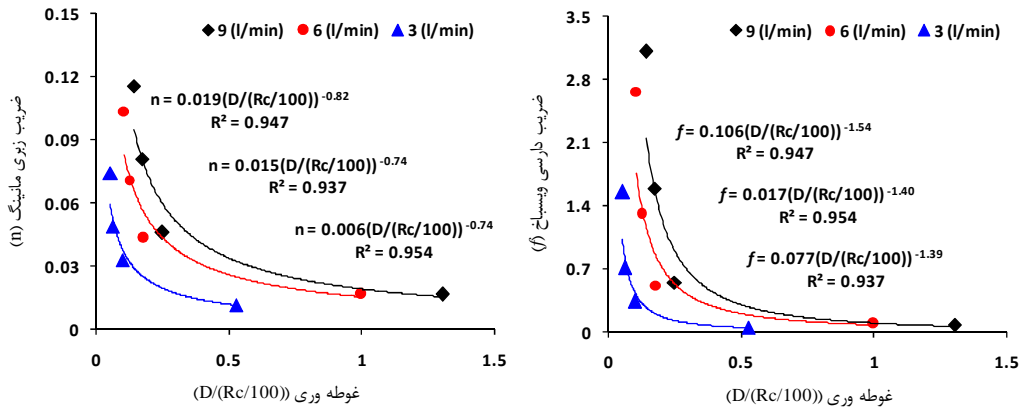
شکل ۶- رابطه بین غوطه‌وری نسبی (D/(Rc/100)) و ضرایب زبری مانینگ و دارسی ویسباخ در دبی‌های مختلف جریان سطحی Figure 6. Relation between relative submergence (D/(Rc/100)) and Manning's and Darcy-Weisbach roughness coefficients in different surface flow discharge
