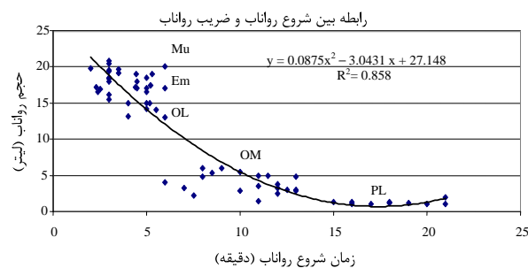
شکل ۹- بررسی رابطه بین زمان شروع رواناب واحدهای کاری با حجم رواناب.
