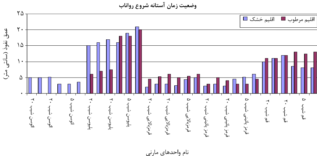
شکل ۸- مقایسه عمق نفوذ آب در واحدهای کاری.
