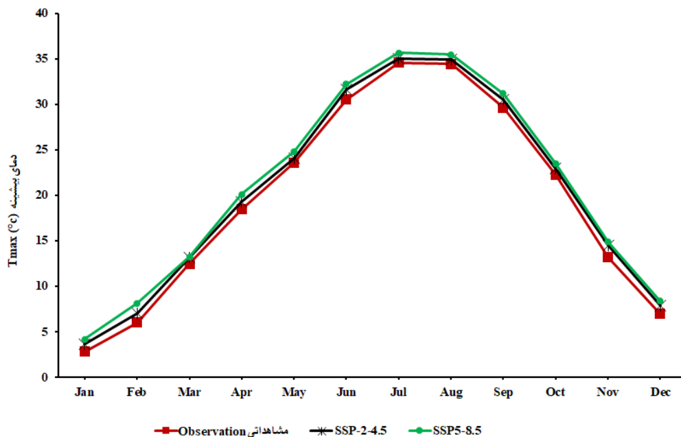
شکل ۴- دمای بیشینه پیش‌نگری شده تحت سناریوهای SSP2-4.5 و SSP5-8.5 در طول دوره (۲۰۷۵-۲۰۵۱) در دشت همدان - بهار Figure 4. The predicted maximum temperature under the SSP2-4.5 and SSP5-8.5 scenarios during the period (2075-2051) in Hamadan-Bahar Plain
