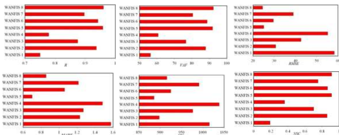
شکل ۹- شاخص‌های آماری برای نتایج شبیه‌سازی بارش توسط مدل‌های WANFIS مختلف Figure 9. Statistical indices for precipitation results simulated by different WANFIS models
