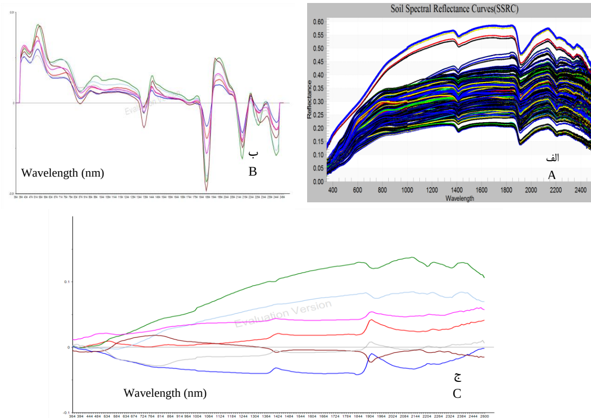
شکل ۲- الف) منحنی‌های بازتابش طیفی (SSRC) نمونه‌های خاک استان مازندران؛ ب) چند طیف نمونه تحت عملیات مشتق اول SG؛ ج) عملیات مرکزگیری طیفی
