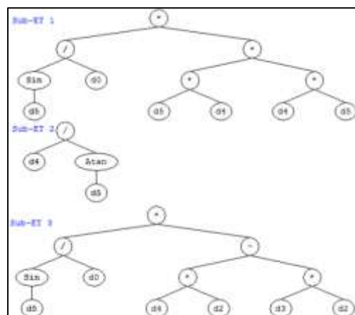
شکل ۷- درخت تجزیه مربوط به رابطه ریاضی مدل بهینه هیبرید موجک-برنامه‌ریزی بیان ژن *d(0), d(1), d(2), d(3), d(4), d(5) و d(6) به‌ترتیب مربوط به متغیرهای فشار هوا، رطوبت هوا، سرعت باد، سرعت تندباد، ارتفاع حداکثر موج و تناوب موج می‌باشد
