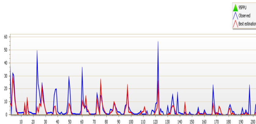
شکل ۴- دبی ماهانه مشاهداتی و شبیه‌سازی‌شده بر حسب متر مکعب بر ثانیه ( m^3 s^{-1} ) توسط مدل طی سال‌های ۱۹۹۶ تا ۲۰۱۲ میلادی Figure 4. Monthly observational and simulated monthly discharge in cubic meters per second ( m^3 s^{-1} ) using SWAT from 1996 to 2012
