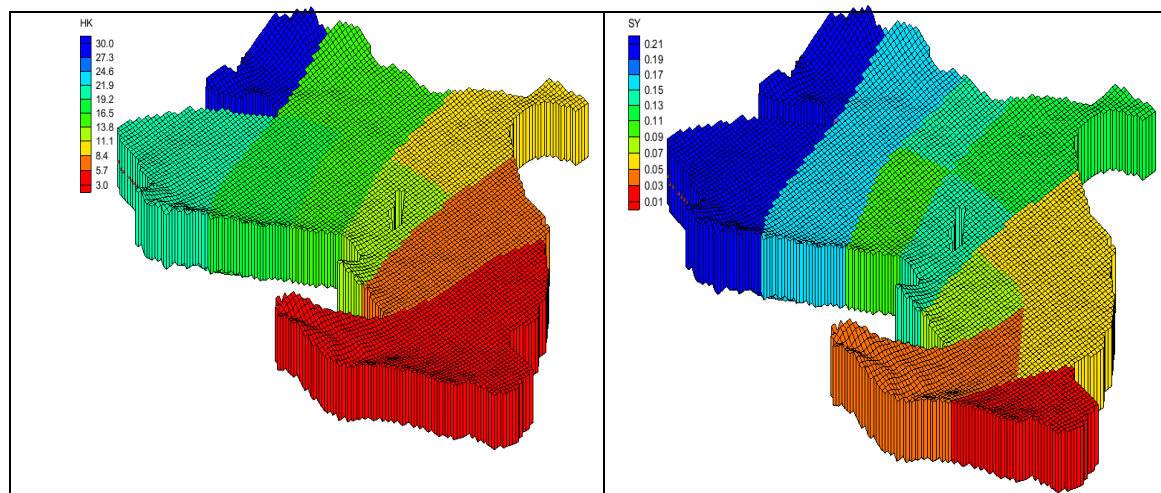
شکل ۶- مقادیر کالیبره شده هدایت هیدرولیکی آبخوان
