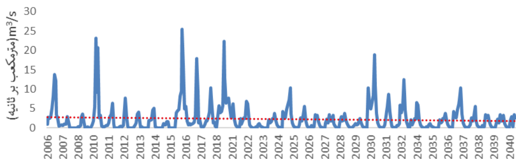
شکل ۱۰- رواناب شبیه‌سازی‌شده رودخانه قره‌سو توسط مدل IHACRES Figure 10. Simulated runoff of the Qarasu River by the IHACRES model
