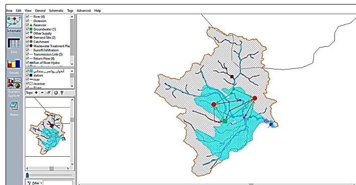
شکل ۴- پیکربندی سامانه منابع آب محدوده روانسر سنجابی در نرم افزار WEAP Figure 4. Configuring the water resources system of the Ravansar-Sinjab area in WEAP software
