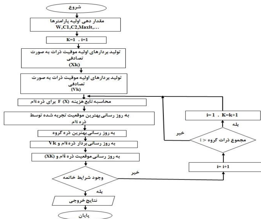
شکل ۵- فلوچارت الگوریتم بهینه‌سازی ازدحام ذرات
