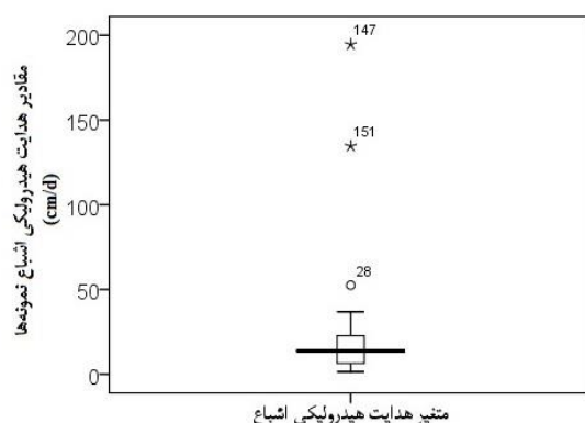
شکل ۱- نمودار جعبه‌ای توزیع هدایت هیدرولیکی اشباع نمونه‌های خاک (سانتیمتر بر روز) Figure 1. Box plot of saturated hydraulic conductivity distribution of the soil samples (ks= saturated hydraulic conductivity (cm/d))
