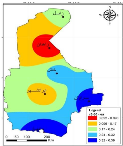
شکل ۱۵- توزیع مکانی همبستگی مابین شاخص‌های پیوند ازدور و شاخص R5-30 Figure 15. Spatial distribution of correlation between teleconnection indices and R5-30
