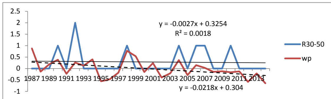
شکل ۵- روند و نوسان شاخص حدی R۳۰-۵۰ نسبت به شاخص WP ایستگاه ابرانشهر Figure 5. Trend and oscillation of R30-50 into WP Iranshahr station
