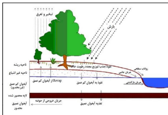
شکل ۳- چرخه هیدرولوژیکی مدل اقتباس از (۲۵) Figure 3. Hydrological cycle model adapted from (25)
