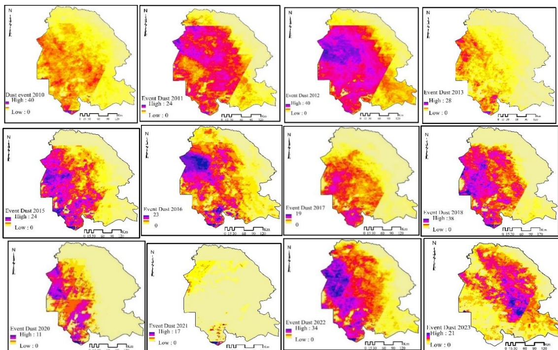
شکل ۶- پراکنده‌ی رویدادهای گرد و غبار در استان خوزستان
