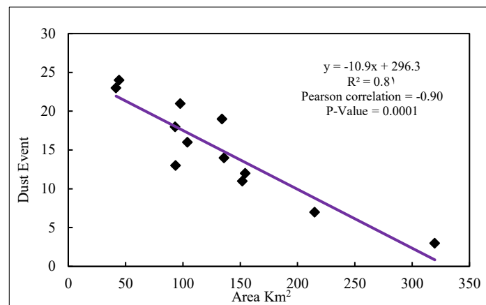
شکل ۵- نمودار تحلیل رگرسیون رویداد گرد و غبار AOD و سطح آبی تالاب شادگان
