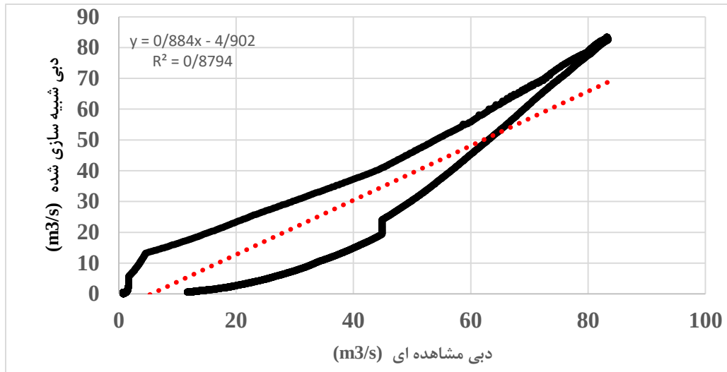
شکل ۱۰- نمودار پراکنش واسنجی سیلاب ۱۰ آذر ۱۳۹۲
