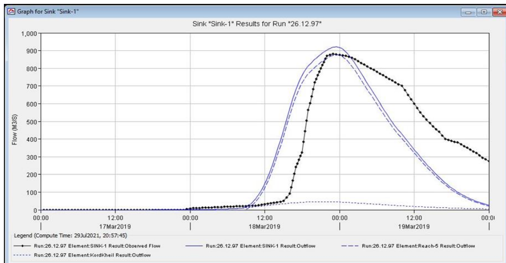
شکل ۱۱- هیدروگراف شبیه‌سازی شده پس از عملیات اعتباریابی در تاریخ ۲۶ اسفند ۱۳۹۷ ایستگاه کردخیل
