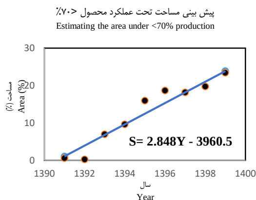
شکل ۴- نمودارهای حاصل از تخمین گر شیب سن و روابط بدست آمده برای نیمه‌ی دوم سال‌های مورد بررسی (S: مساحت تحت هر محدوده عملکرد (% و Y: سال)
