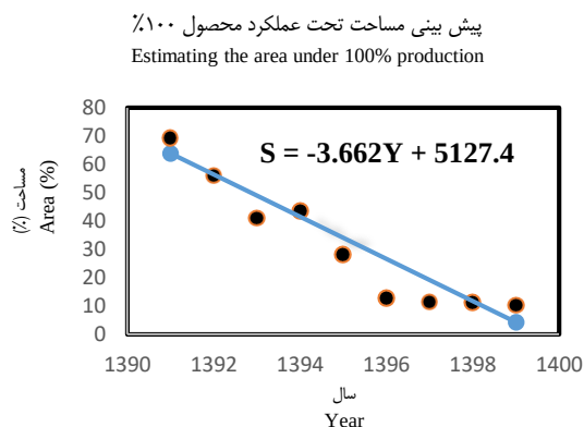
شکل ۳- نمودارهای حاصل از تخمین گر شیب سن و روابط بدست آمده برای نیمه‌ی اول سال‌های مورد بررسی (S: مساحت تحت هر محدوده عملکرد (% و Y: سال)
