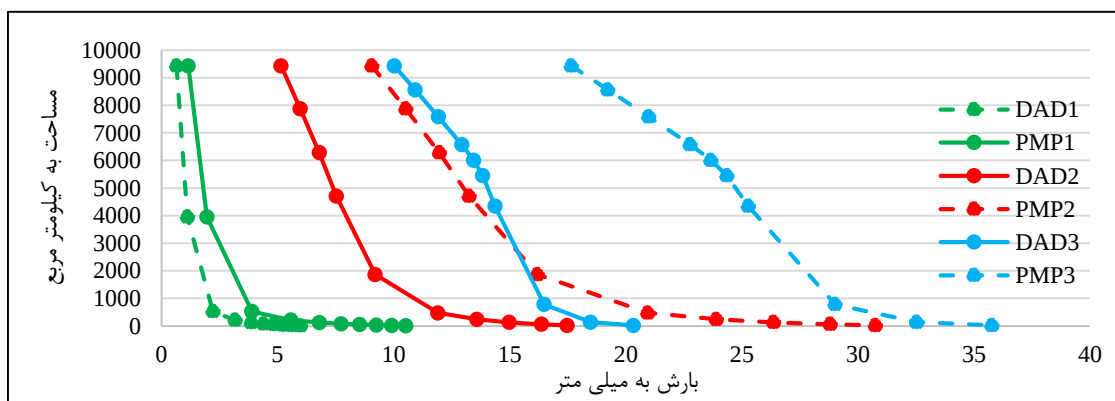
شکل ۹- منحنی‌های عمق - سطح - تداوم و حداکثر بارش محتمل ۱ الی ۳ روزه Figure 9. Depth - area - duration and probable maximum precipitation 1 to 3 days
