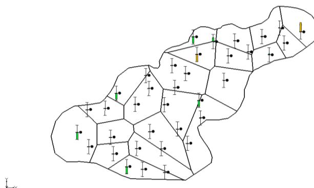
شکل ۴- وضعیت سطح آب شبیه‌سازی شده و اندازه‌گیری شده در پیزومترهای منطقه مورد مطالعه برای حالت پایدار Figure 4. Simulated and measured water level status in piezometers of the study area for steady state
