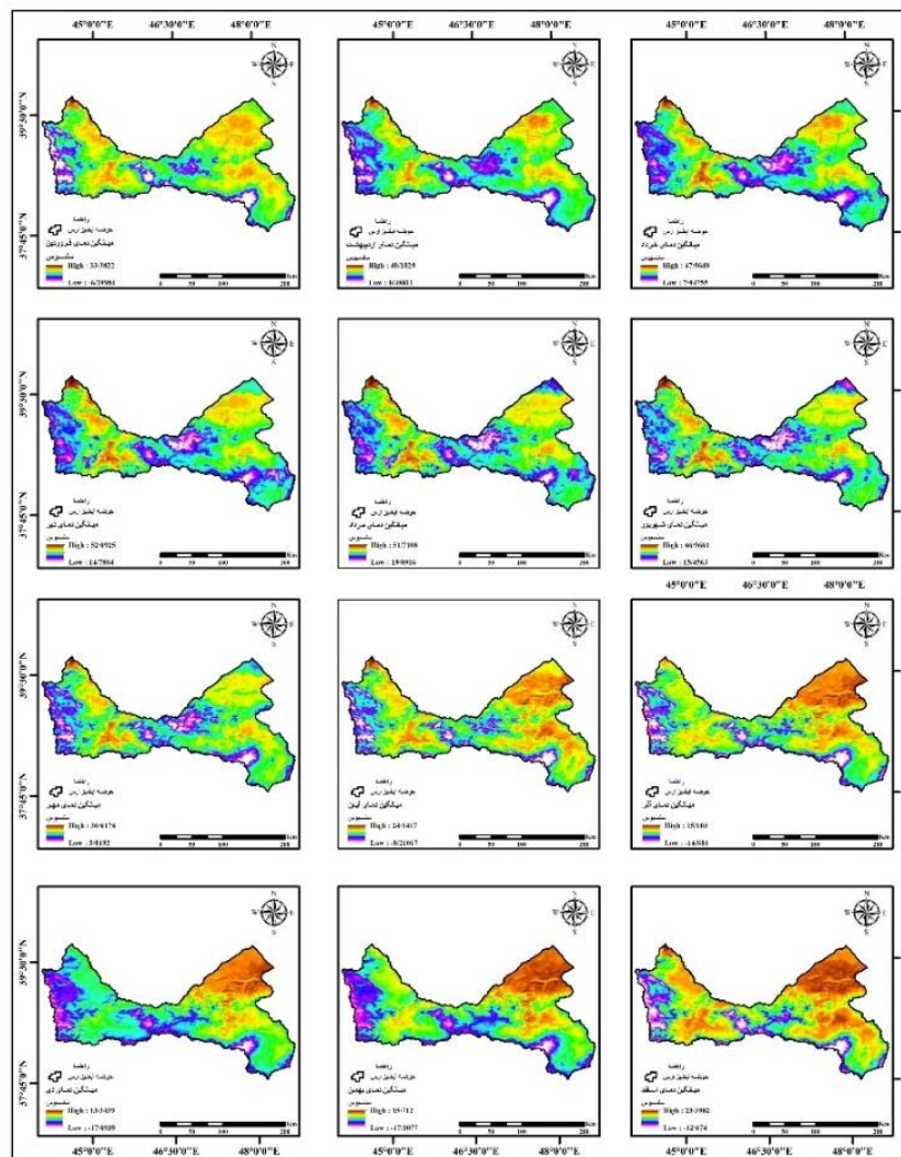
شکل ۵- میانگین ماهانه دمای سطح زمین در حوزه آبخیز ارس
