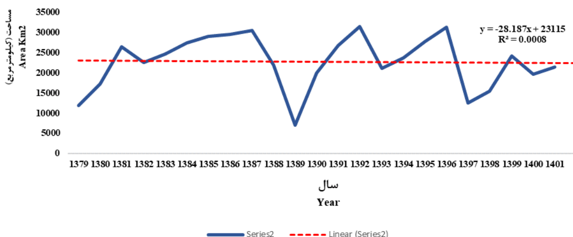
شکل ۱۸- تغییرات سالانه پوشش برف (NDSI) در حوزه آبخیز ارس (کیلومتر مربع) Figure 18. Annual snow cover changes (NDSI) in the Aras Basin (Km²)
