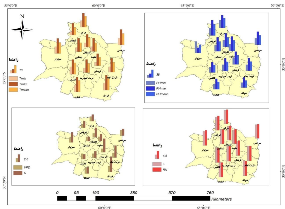
شکل ۲- متوسط پارامترهای هواشناسی مورد استفاده در تعیین تبخیر و تعرق فائو پنمن مانتیث در مناطق مورد مطالعه Figure 2. The average of meteorological parameters used in determination of FAO- Penman - Monteith evapotranspiration across the study areas
