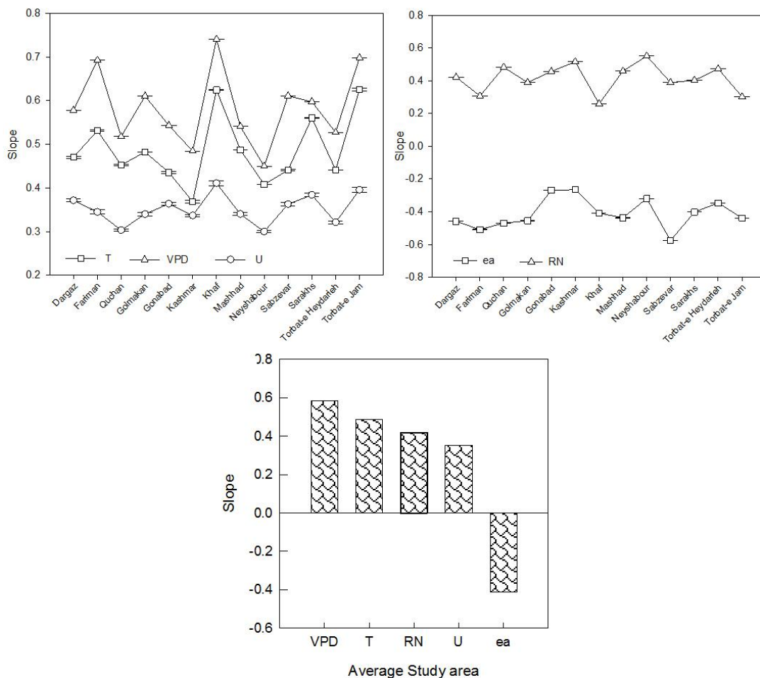
شکل ۵- شیب درصد تغییرات تبخیر و تعرق فائو پنمن و انحراف معیار خطای شیب نسبت به تغییر پارامترهای هواشناسی در مناطق مورد مطالعه و متوسط شیب در کل استان خراسان رضوی
