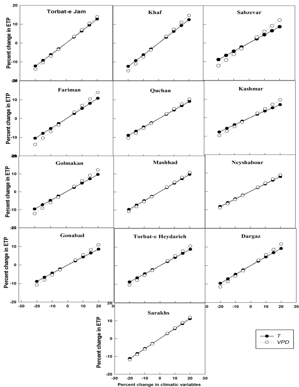
شکل ۳- درصد تغییرات تبخیر و تعرق فائو پنمن ماتیت نسبت به تغییر پارامترهای هواشناسی درجه حرارت و کمبود فشار بخار Figure 3. The percent change of FAO- Penman- Monteith evapotranspiration method to the meteorological parameters (temperature and vapor pressure deficit)
