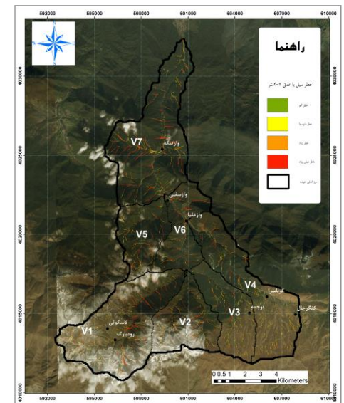
شکل ۱۲- نقشه خطر سیلاب ۲۵ ساله حوضه آبخیز وازرود Figure 12. 25-year flood risk map of Vazrood watershed
