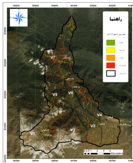
شکل ۱۴- نقشه خطر سیلاب ۱۰۰ ساله حوزه آبخیز وازرود
