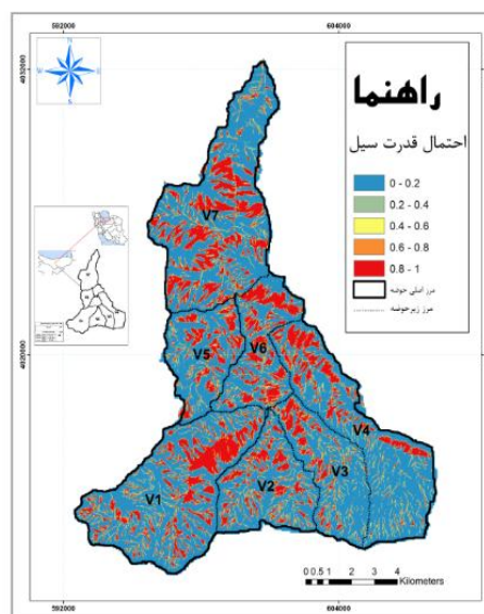
شکل ۹- نقشه احتمالاتی شاخص قدرت رودخانه حوضه آبخیز وازرود (۲۴) Figure 9. Probability Map of The Power Index of The Vazrood Watershed (24)
