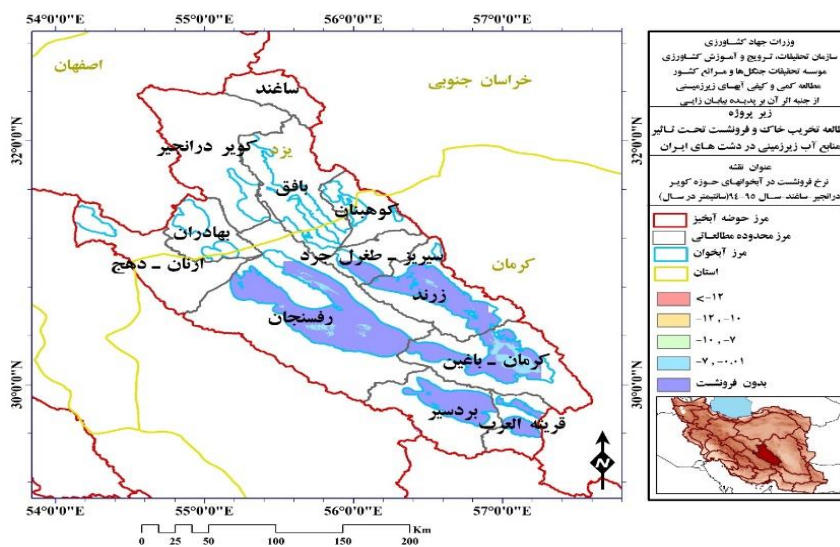
شکل ۱۰- نرخ فرونشست در آبخوان محدوده‌های مطالعاتی حوزه آبریز کویر درانجیر Figure 10. The subsidence rate in the aquifer of the study areas of the Daranjir watershed
