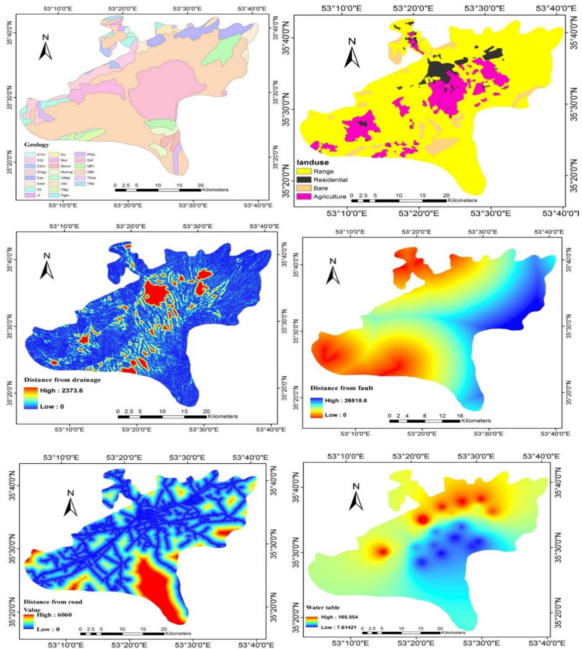
ادامه شکل ۲- نقشه‌های عوامل مؤثر بر فرونشست زمین در دشت سمنان Continued figure 2. Conditioning factors of land subsidence in Semnan plain
